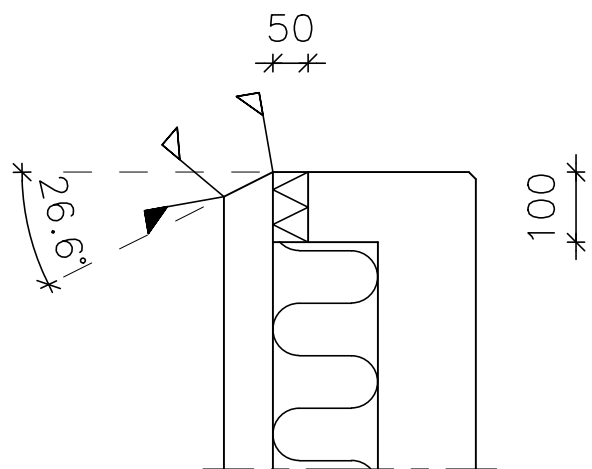
LODRET SNIT
